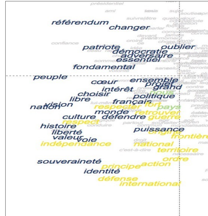
MLP
