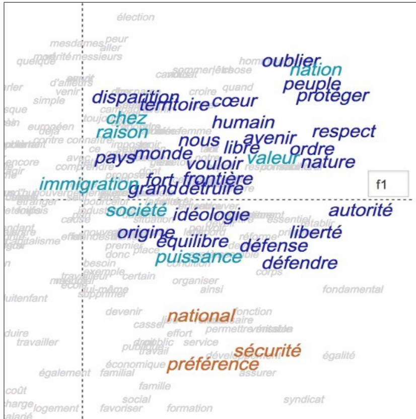
JMLP
